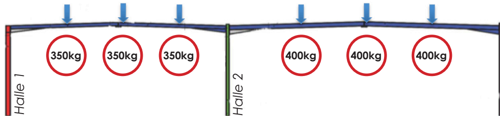
Cas n°3 Halle 1 : charges ponctuelles de 350kg situées mi-longueur de la traverse et au faitage. Halle 2 : charges ponctuelles de 400kg situées mi-longueur de la traverse et au faitage.
