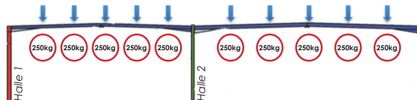
Cas n°4 Halle 1 : charges ponctuelles de 250kg écartées de 2,45m les unes des autres. Halle 2 : charges ponctuelles de 250kg écartées de 2,45m les unes des autres.
