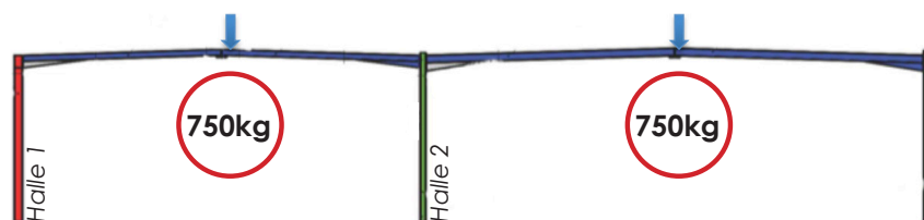
Cas n°1 Charge ponctuelle de 750kg au niveau du faitage.
